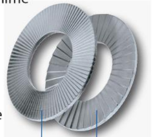
radyal dişler kamalı yüzeyler
